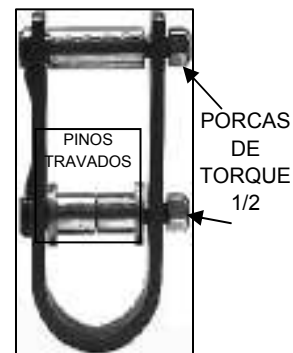
U-10.023 = COD. 789 PAR C/ BUCHAS AÇO E PINOS PARA LUBRIFICAÇÃO REFORÇADO - C/CHAPA 5/16 E MAIOR DISTANCIA ENTRE FUIROS
