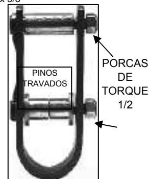
U-10.023 = COD. 789 PAR C/ BUCHAS AÇO E PINOS PARA LUBRIFICAÇÃO REFORÇADO E COM MAIOR DISTANCIA ENTRE FUROS
